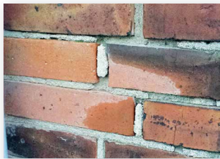
Offene Fugen am Verblendstein
